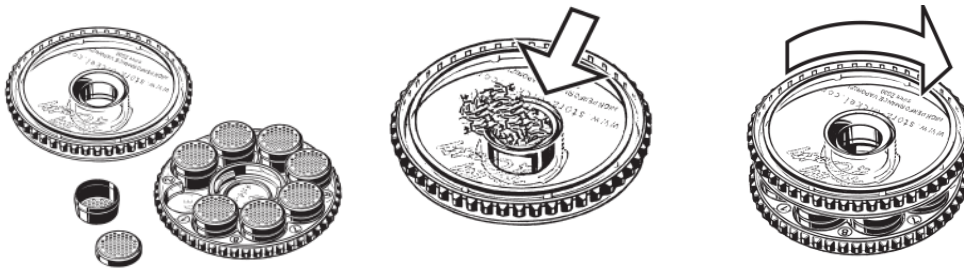
ΚΑΦΟΥΛΑ ΔΟΣΟΛΟΓΙΑΣ ΚΑΤΑ ΤΟ ΓΕΜΙΣΜΑ ΜΕ ΤΟ ΚΑΠΑΚΙ ΤΟΥ ΓΕΜΙΣΤΗΡΑ (ΧΟΑΝΗ) ΚΑΙ ΤΟ- ΠΟΘΕΤΗΣΗ ΤΟΥ ΚΑΠΑΚΙΟΥ ΣΤΟ ΓΕΜΙΣΤΗΡΑ
